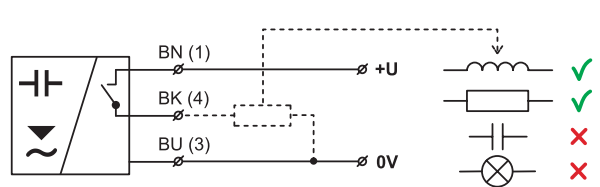
Zapojení snímače s výstupem typu PNP (varianta „P“)
