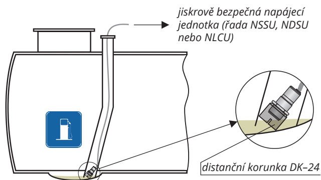
Použití CPS k indikaci přítomnosti kapaliny v meziplášťovém prostoru
