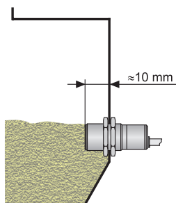
Snímání sypkých materiálů v zásobníku
