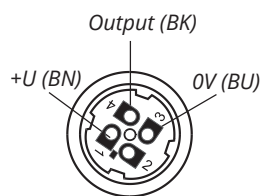
Vnitřní pohled na konektorovou zásuvku
