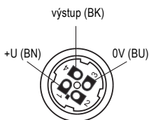
Obr. 20: Vnitřní pohled na konektorovou zásuvku
