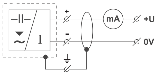
Obr. 2: Schéma připojení hladinoměru s proudovým výstupem CLM-70_--_I
