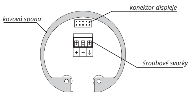
Obr. 3: Vnitřní pohled na šroubové svorky hladinoměru s proudovým výstupem CLM-70_--_I
