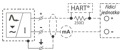
obr. 13: Schéma zapojení hladinoměru s proudovým výstupem ARLM-70 __-I
