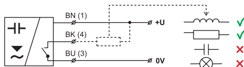
Obr. 7: zapojení snímače s výstupem typu NPN (varianta „N“)
