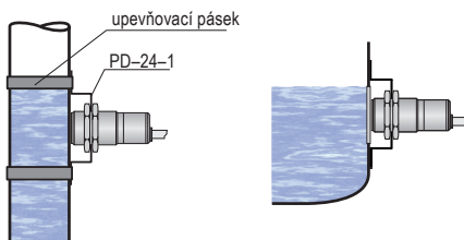
Obr. 4: Aplikace snímačů CPS na stavoznaky a průhledítka
