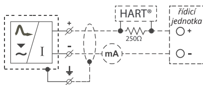
obr. 13: Schéma zapojení hladinoměru s proudovým výstupem ARLM-70_--_-I
