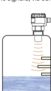
obr. 5: Falešná ozvěna od překážek v nádrži
