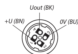
Obr. 24: Vnitřní pohled na konektorovou zásuvku (varianta "C")
