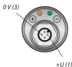
Obr. 23: Připojovací schéma a vnitřní pohled na konektor hladinoměru DLM (varianta - I)
