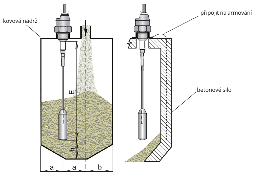
Obr. 22: Instalace hladinoměrů s lanovou elektrodou
