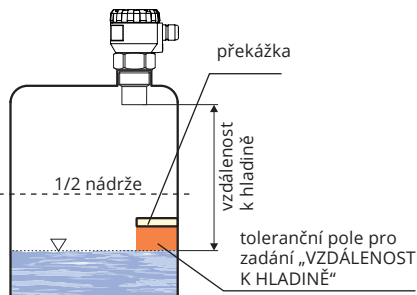
Obr. 21: Úroveň hladiny pro zadání hodnoty „Set level distance“
