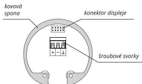
Vnitřní pohled na šroubové svorky hladinoměru s proudovým výstupem GRLM-70_--I
