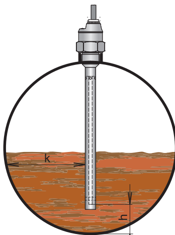
Obr. 3: Instalace hladinoměří s referenční trubkou
